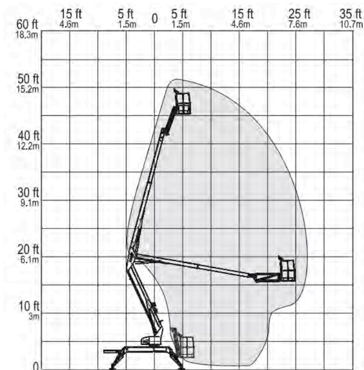
NACELLE REMORQUABLE MODÈLE 4527A
