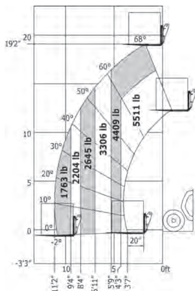
CHARIOT TÉLESCOPIQUE 19' MODÈLE MT-625
