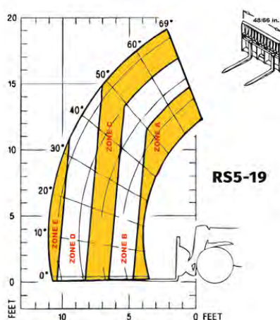
CHARIOT TÉLESCOPIQUE 19' MODÈLE RS 5-19
