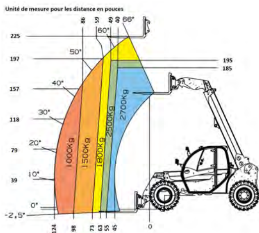
CHARIOT TÉLESCOPIQUE 19' MODÈLE TH 627
