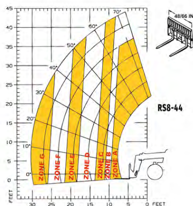
CHARIOT TÉLESCOPIQUE 44' MODÈLE RS 8-44
