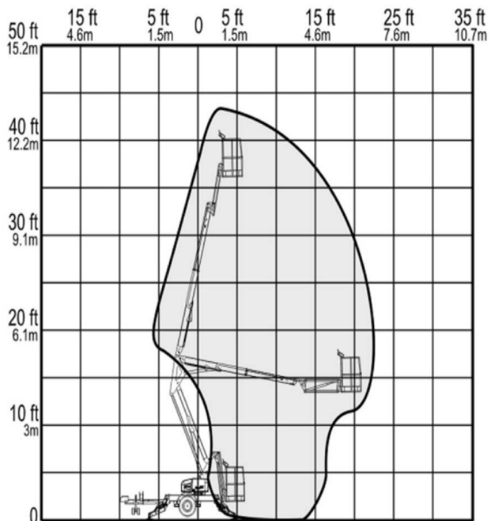
NACELLE REMORQUABLE MODÈLE 3522A
